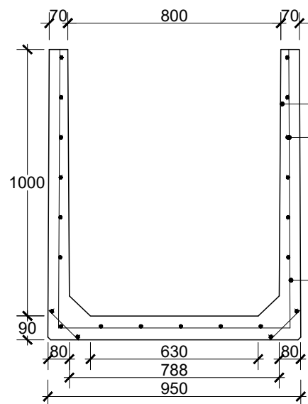
DETAIL PENULANGAN SKALA 1 : 10
