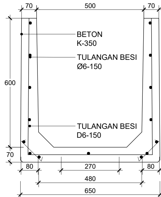
DETAIL PENULANGAN SKALA 1 : 10
