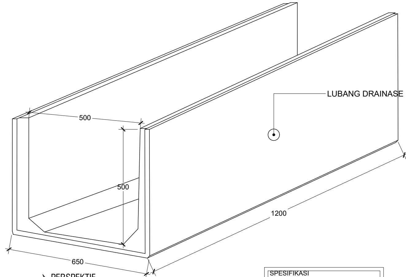
PERSPEKTIF SKALA 1 : 10
