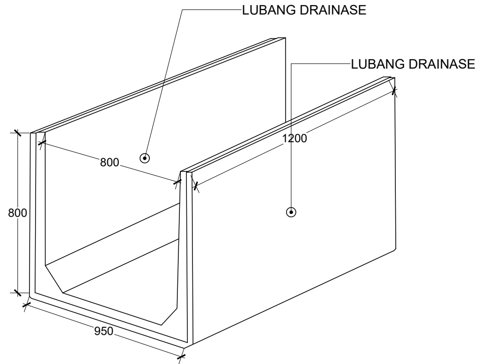
PERSPEKTIF SKALA 1 : 10
