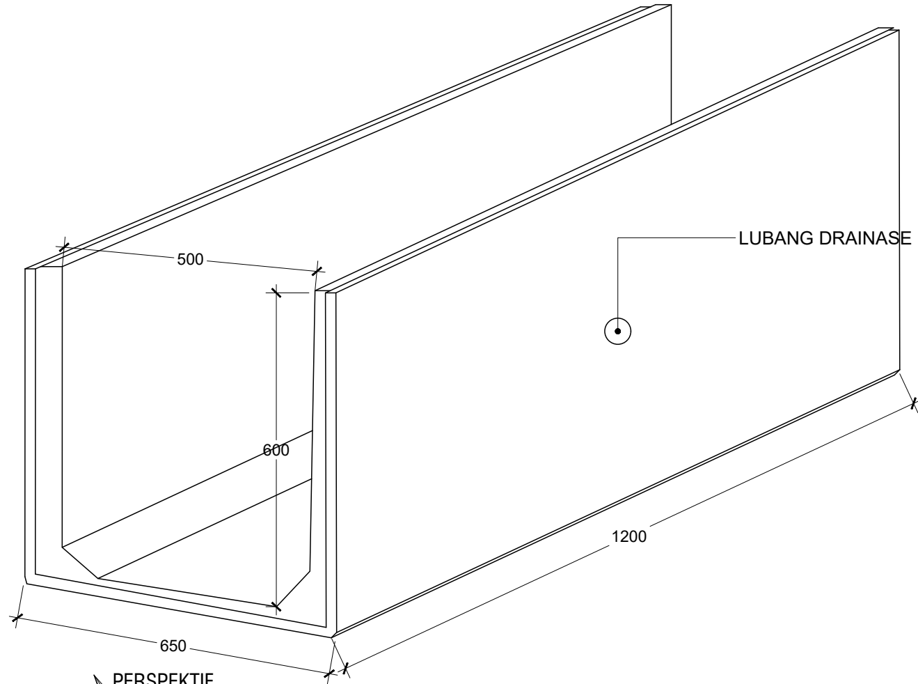
PERSPEKTIF SKALA 1 : 10
