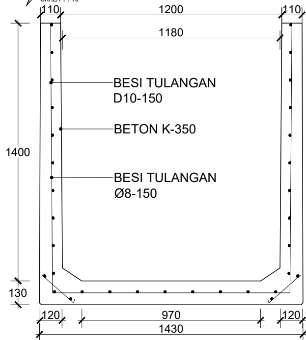
DETAIL PENULANGAN
