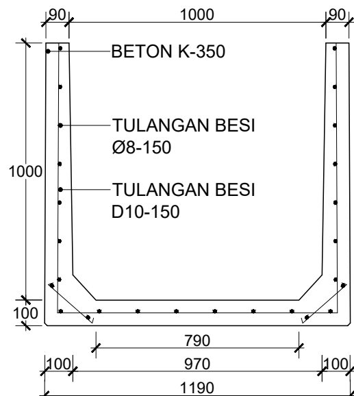
DETAIL PENULANGAN
