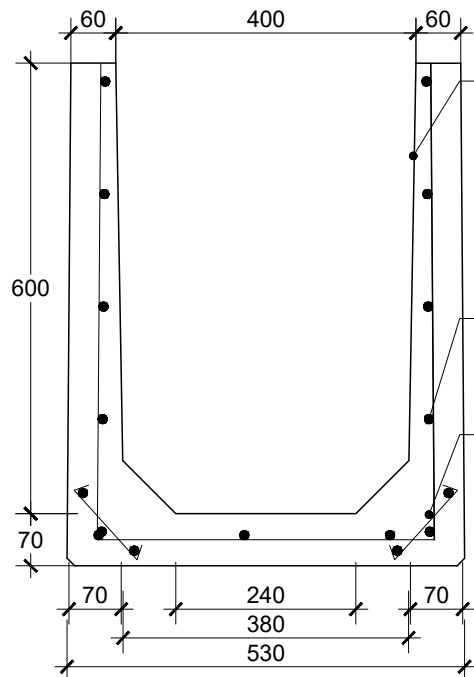
DETAIL PENULANGAN SKALA 1 : 10
