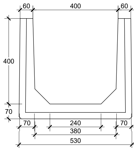
TAMPAK DEPAN U-DITCH 400 X 400 SKALA 1 : 10
