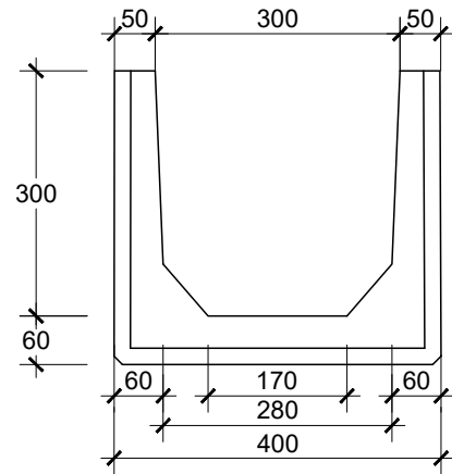
TAMPAK DEPAN U-DITCH 300 X 300 SKALA 1 : 10
