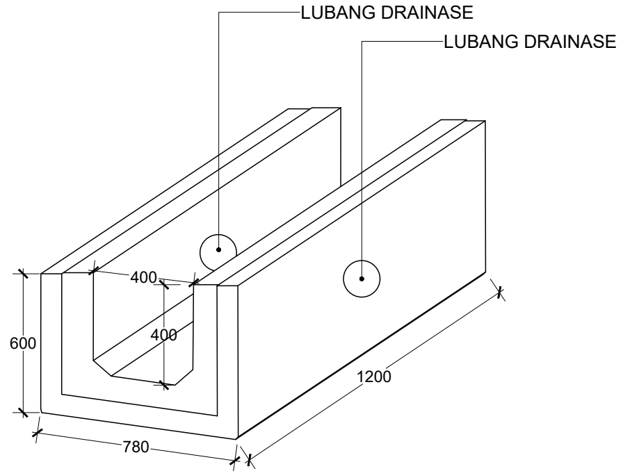
PERSPEKTIF SKALA 1 : 10
