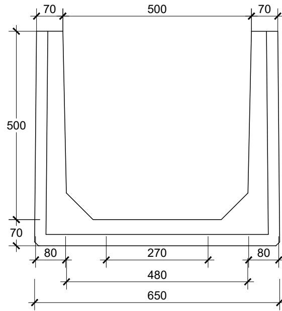
TAMPAK DEPAN U-DITCH 500 X 500 SKALA 1 : 10
