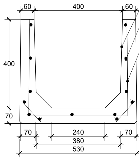
DETAIL PENULANGAN SKALA 1 : 10
