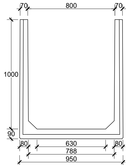
TAMPAK DEPAN U-DITCH 800 X 1000 SKALA 1 : 10
