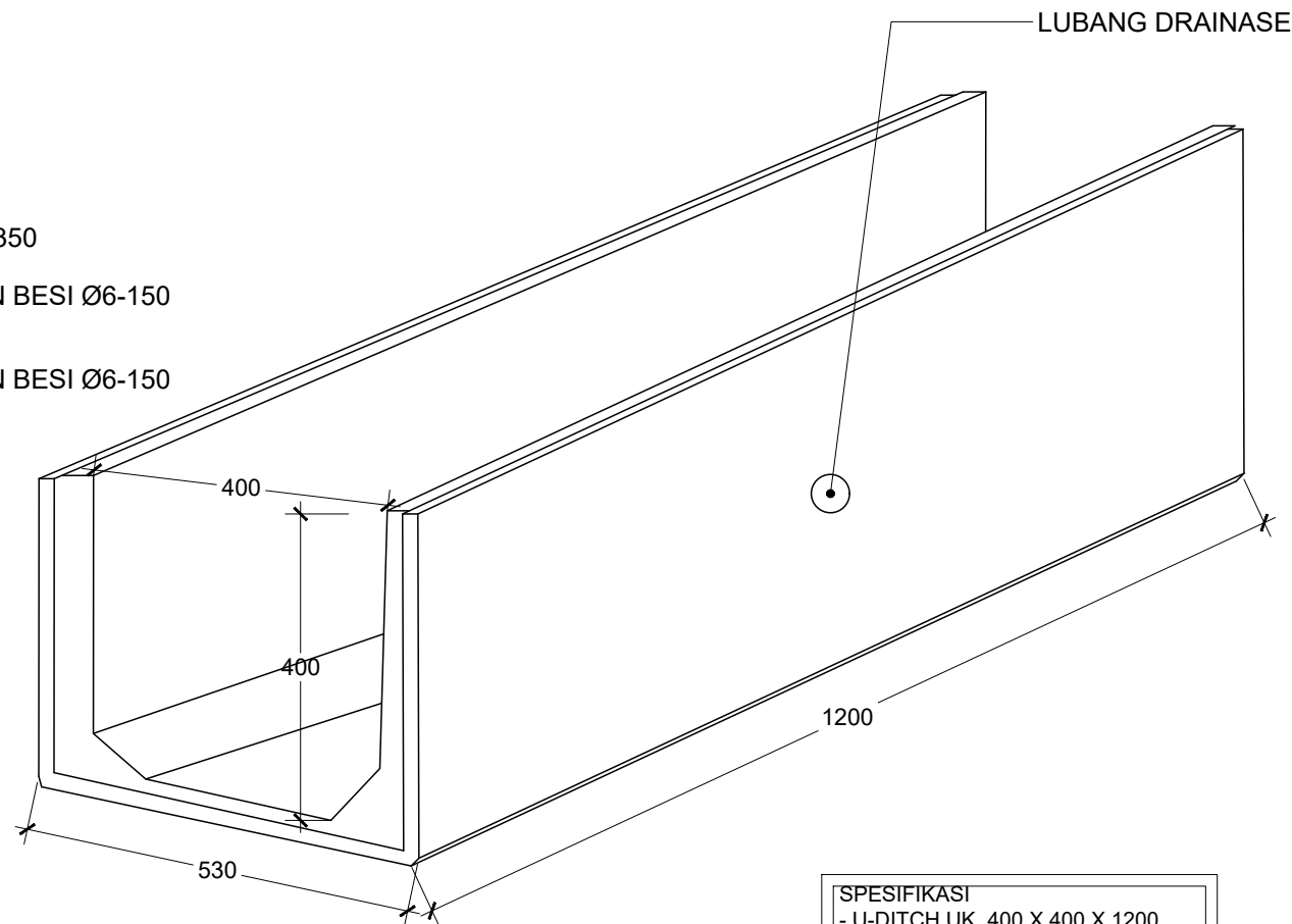
PERSPEKTIF SKALA 1 : 10
