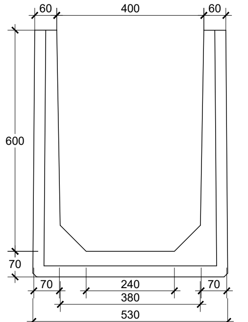
TAMPAK DEPAN U-DITCH 400 X 600 SKALA 1 : 10
