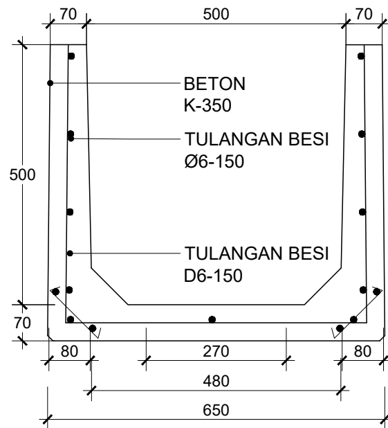
DETAIL PENULANGAN SKALA 1 : 10
