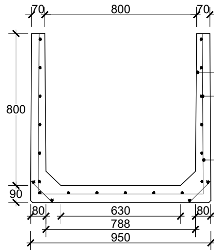
DETAIL PENULANGAN SKALA 1 : 10
