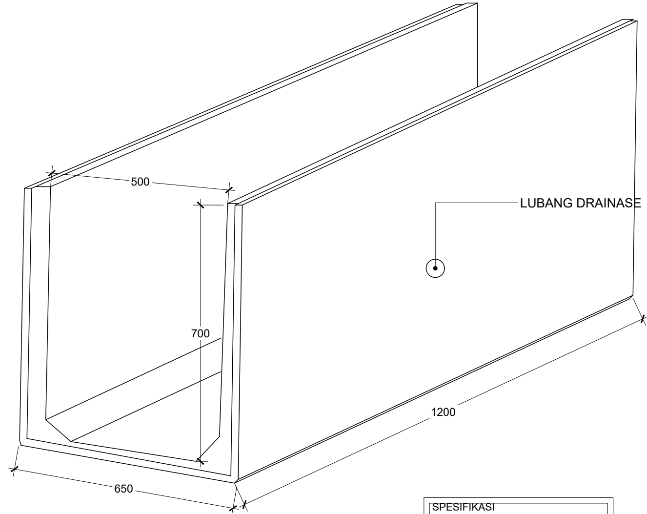
PERSPEKTIF SKALA 1 : 10
