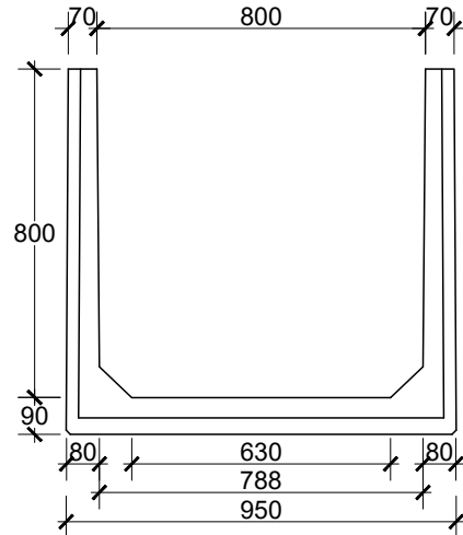
TAMPAK DEPAN U-DITCH 800 X 800 SKALA 1 : 10
