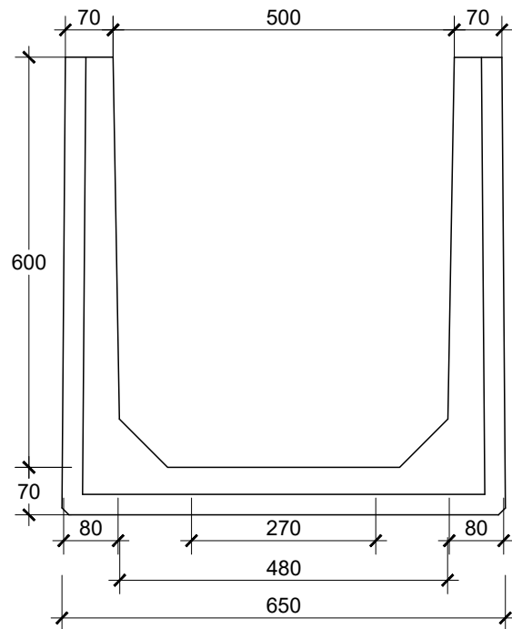
TAMPAK DEPAN U-DITCH 500 X 600 SKALA 1 : 10
