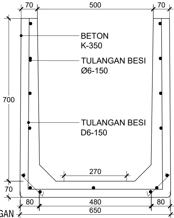
TAMPAK DEPAN U-DITCH 500 X 700 SKALA 1 : 10
