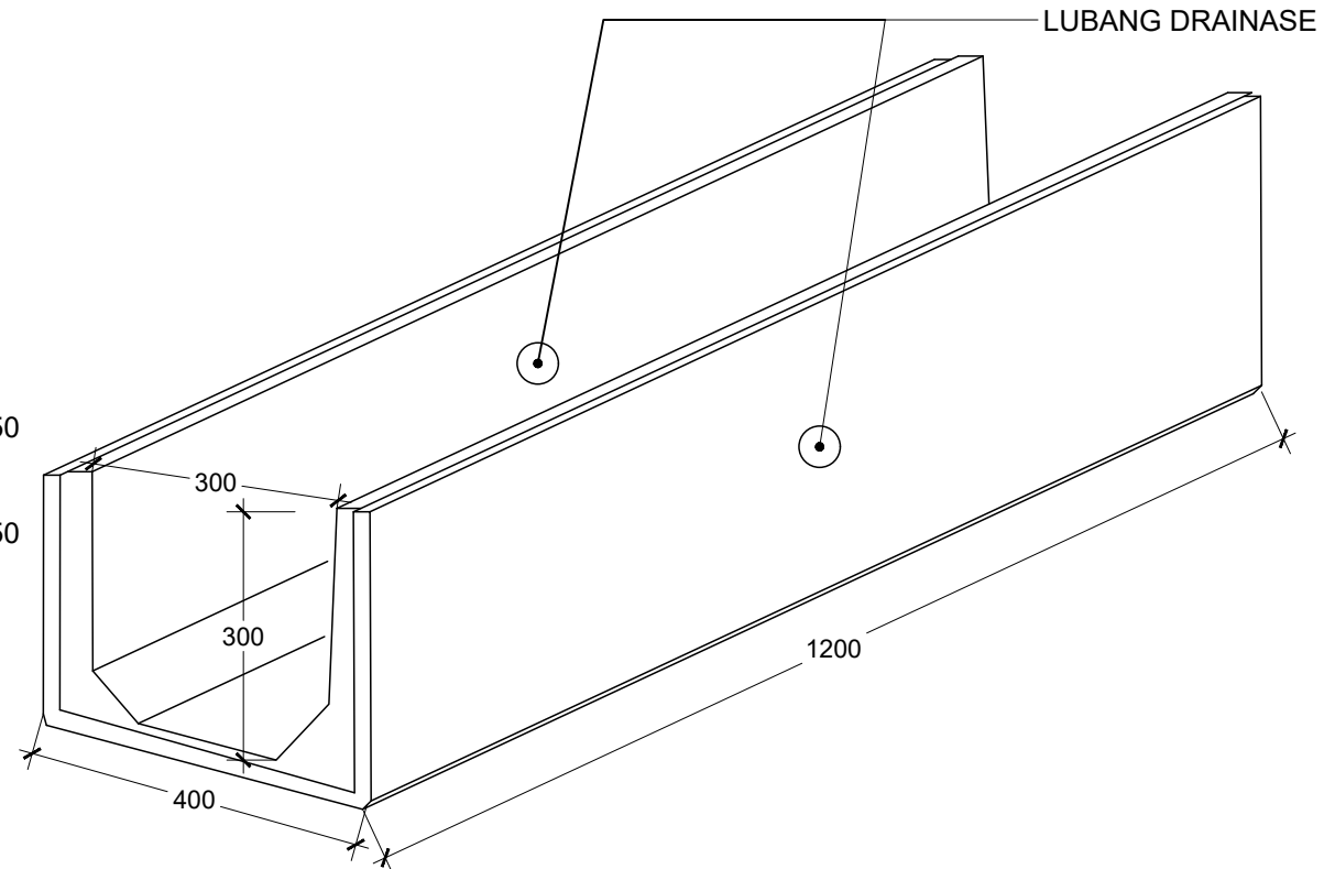
PERSPEKTIF SKALA 1 : 10
