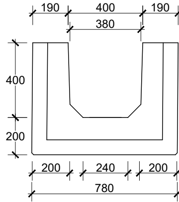
TAMPAK DEPAN U-DITCH 400 X 400 DOUBLE SKALA 1 : 10
