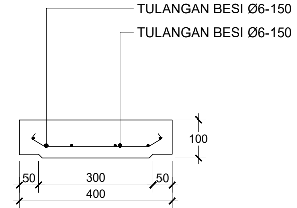
DETAIL PENULANGAN SKALA 1 : 10
