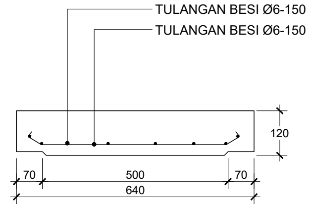
DETAIL PENULANGAN SKALA 1 : 10
