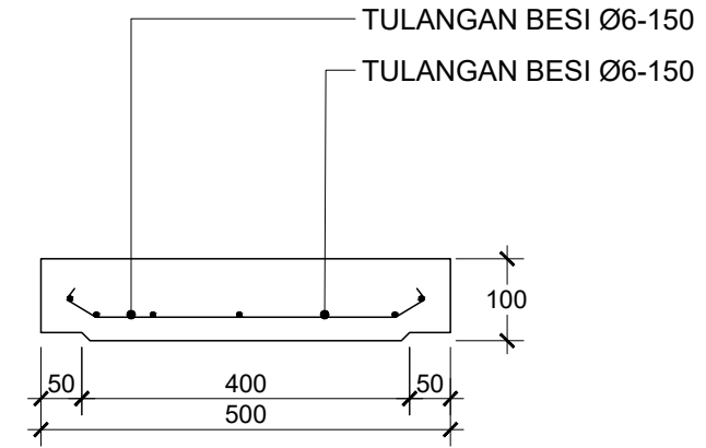
DETAIL PENULANGAN SKALA 1 : 10
