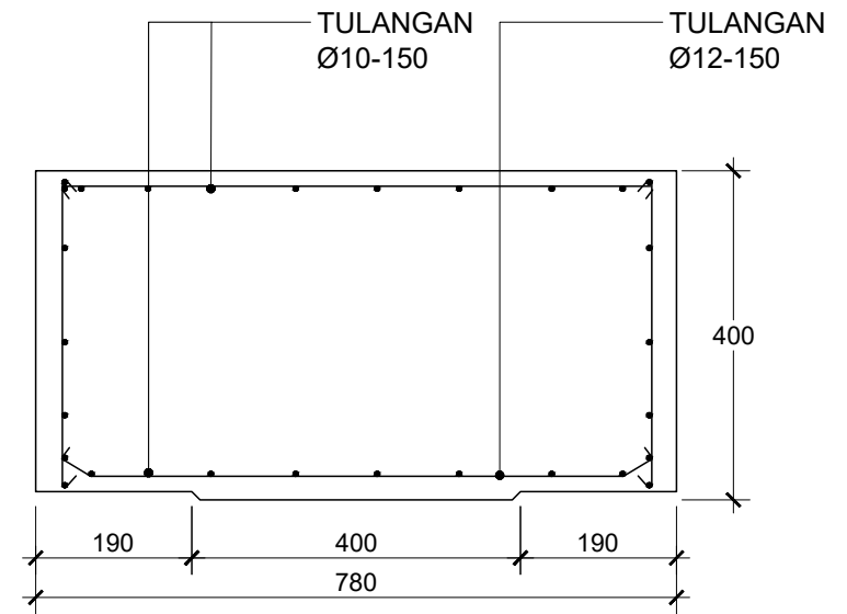
DETAIL PENULANGAN SKALA 1 : 10
