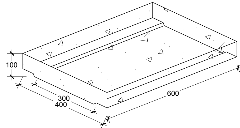
PERSPEKTIF SKALA 1 : 10
