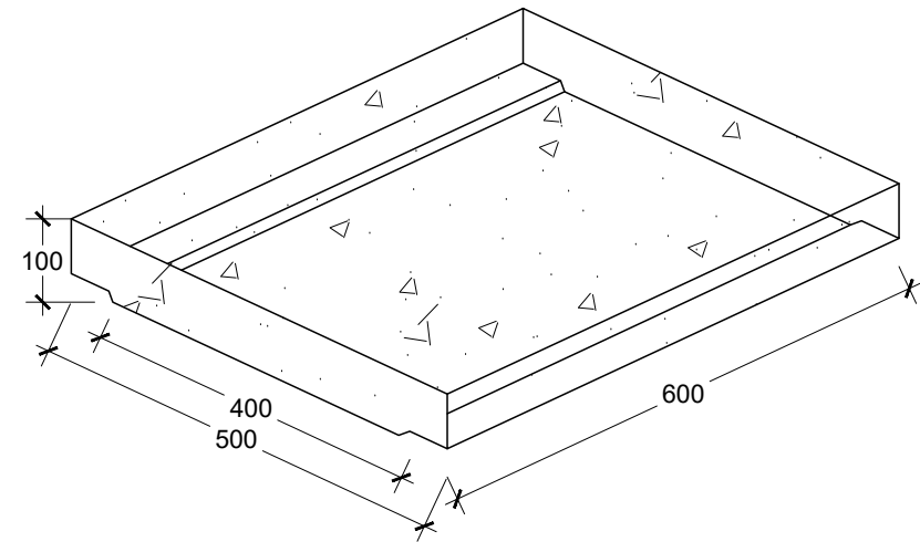
PERSPEKTIF SKALA 1 : 10
