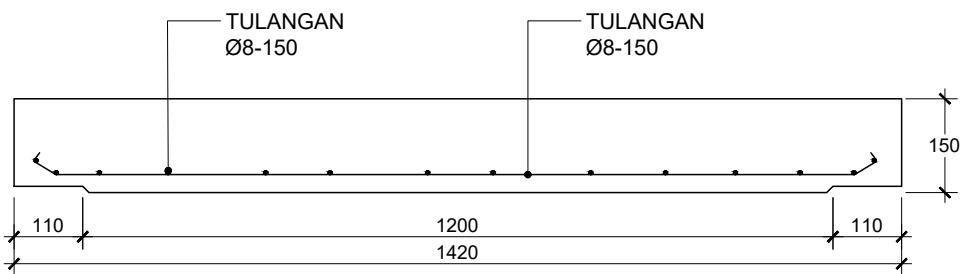
DETAIL PENULANGAN SKALA 1 : 10
