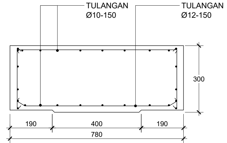
DETAIL PENULANGAN SKALA 1 : 10
