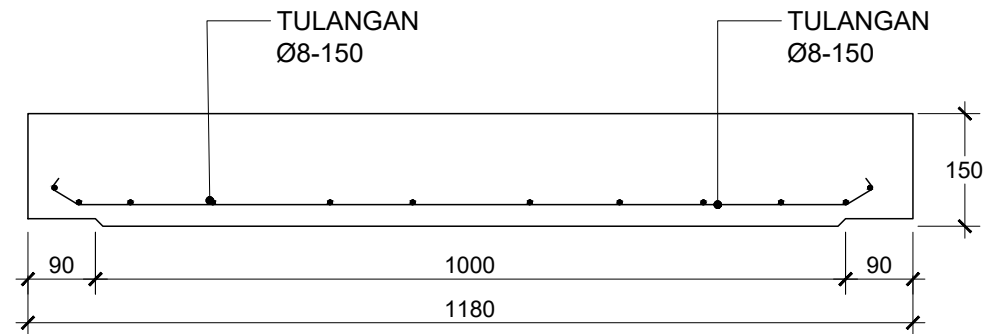
DETAIL PENULANGAN SKALA 1 : 10
