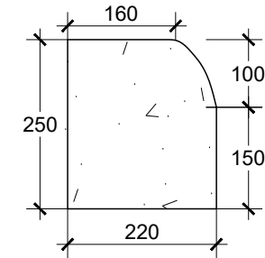
TAMPAK SAMPING KANSTEIN TYPE C T. 25 CM SKALA 1 : 10
