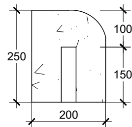
TAMPAK SAMPUNG KANSTEIN TYPE A SKALA 1 : 10
