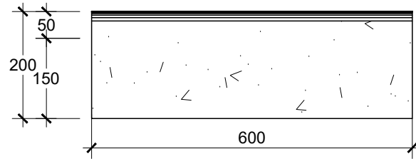
TAMPAK ATAS KANSTEIN TYPE C T. 25 cm SKALA 1 : 10
