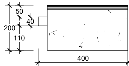
TAMPAK ATAS KANSTEIN TYPE A SKALA 1 : 10
