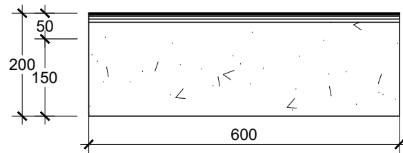
TAMPAK ATAS KANSTEIN TYPE TYPE C T. 30 SKALA 1 : 10
