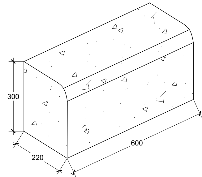
PERSPEKTIF SKALA 1 : 10
