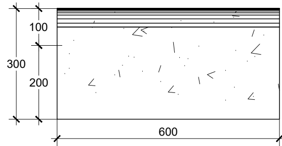
TAMPAK DEPAN KANSTEIN TYPE C T. 30 SKALA 1 : 10
