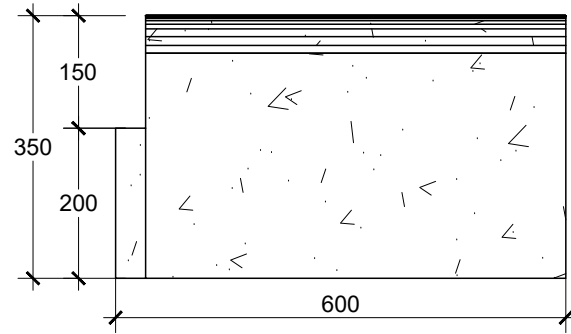
TAMPAK DEPAN KANSTEIN TYPE B SKALA 1 : 10
