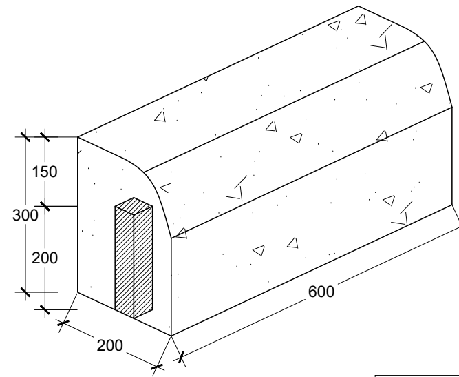
PERSPEKTIF SKALA 1 : 10
