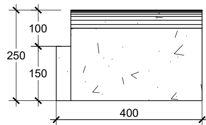
TAMPAK DEPAN KANSTEIN TYPE A SKALA 1 : 10
