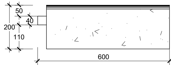
TAMPAK ATAS KANSTEIN TYPE B SKALA 1 : 10
