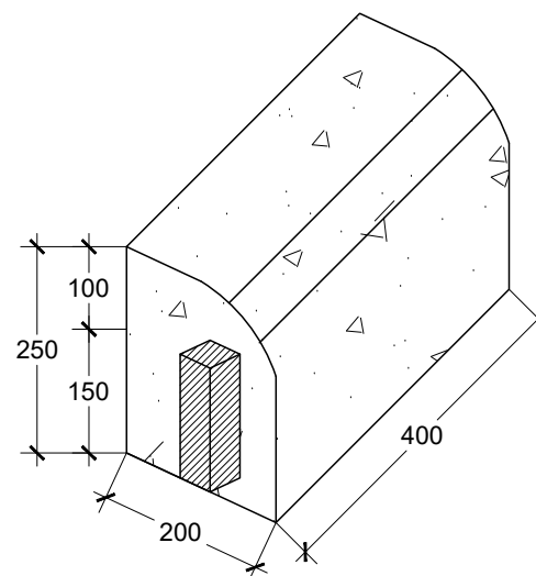
PERSPEKTIF SKALA 1 : 10
