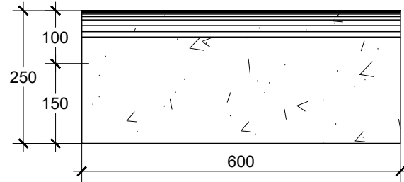
TAMPAK DEPAN KANSTEIN TYPE C T. 25 CM SKALA 1 : 10
